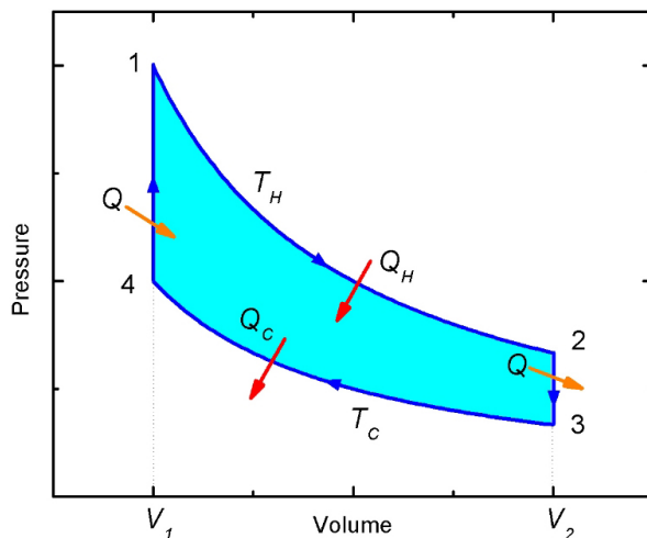
73. ábra. Stirling motor pV diagramon ábrázolva
