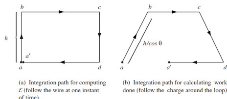
105. ábra. A húzó erő és a töltések mozgása a vezetőben
