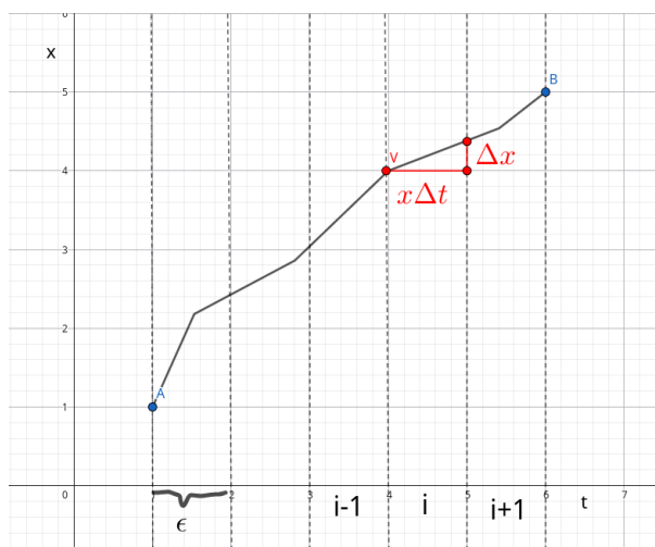
9. ábra. Diszkretizáció
