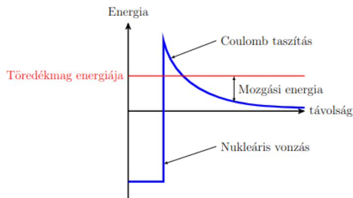
207. ábra. A maghasadás potenciálgátja.
