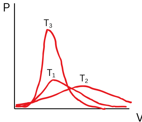
56. ábra. Kinetikus gázelmélet részecske sebesség eloszlása
