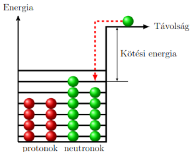
208. ábra. Neutron befogódás és maghasadás.
