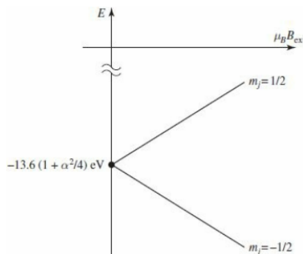
187. ábra. A gyenge Zeeman-effektus hatása a Hidrogén atom energiáinak felhasadására. Az alapállapot két részre szakad m_j = \pm 1/2 szerint.
