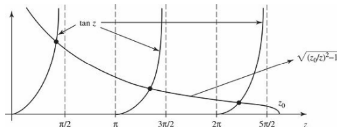
26. ábra. Véges potenciálvölgy megengedett energiák grafikus megoldása z_0 = 8 esetén
