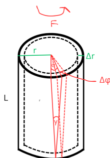
38. ábra. Csavarás
