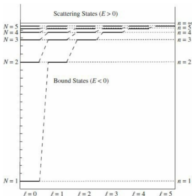
31. ábra. A Hidrogén atom energiaszintjei és hullámfüggvényei; n = 1 az alapállapot E_1 = -13.6 eV energiával; Végtelen számú állapot fér be n = 5 és n = \infty közé; E_\infty = 0 választja el a kötött és szabad állapotokat.
