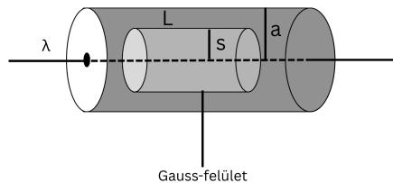
97. ábra. Hosszú vékony vezeték szigetelővel körbevéve
