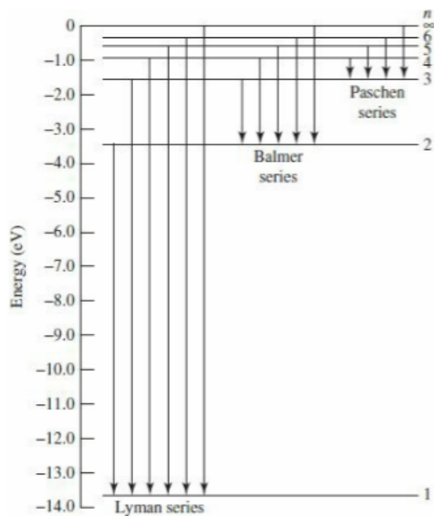
33. ábra. A Hidrogén atom spektrumának Energia szintjei és átmenetei.
