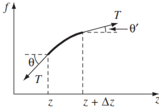
115. ábra. Kötél hulláma
