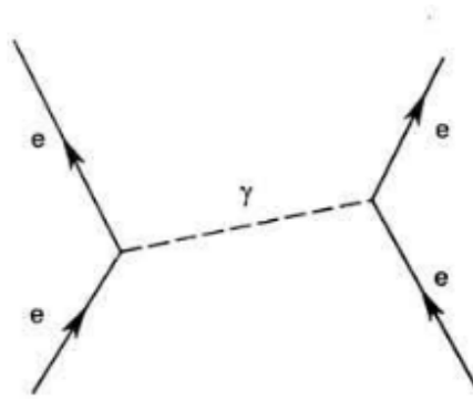
224. ábra. Az erők kicserélődési képének szemléltetése Feynman-gráffal. Jelen esetben elektron szóródik eelektronon és a kölcsönhatást egy \gamma kvantum közvetíti.
