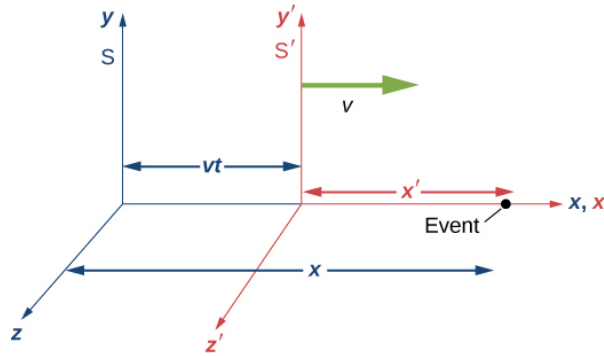
Figure 6: Lorentz transzformáció
