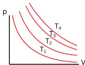
54. ábra. Ideális gáz állapotfelülete a pV térben
