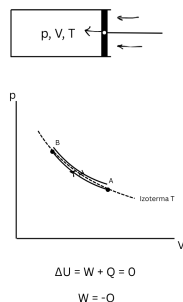
63. ábra. Reverzibilis folyamat egy dugattyús hengerben
