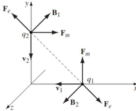
113. ábra. Mozgó töltések ütközése
