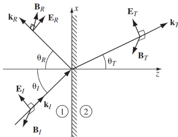
121. ábra. Beesési szög és törési szög
