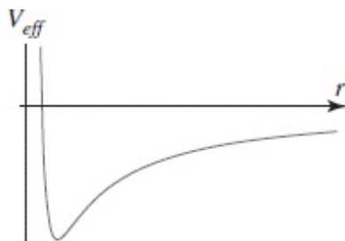
30. ábra. A Hidrogén atom effektív potenciálja
