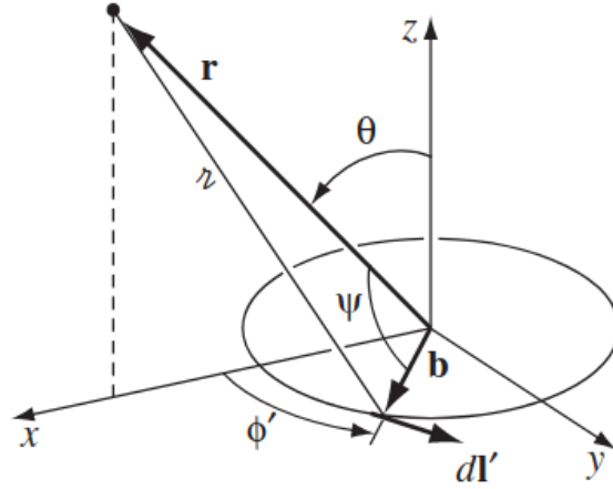
129. ábra. Mágneses dipólsugárzás geometriája
