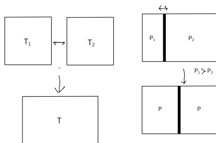
62. ábra. Néhány irreverzibilis folyamat schematikus ábrázolása
