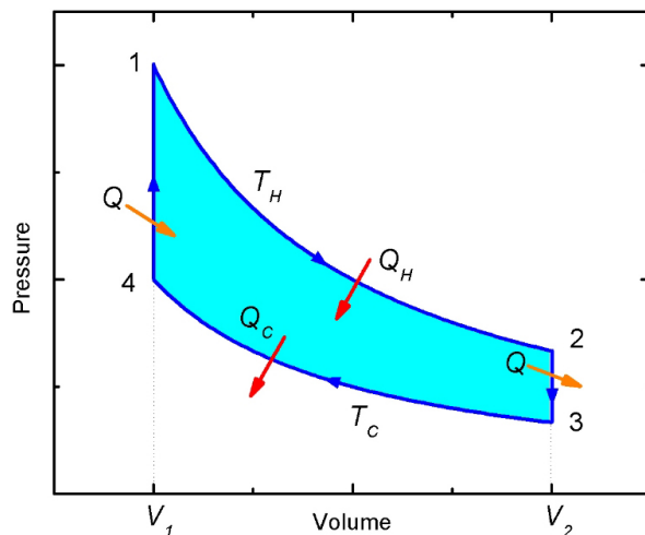
72. ábra. Stirling motor pV diagramon ábrázolva
