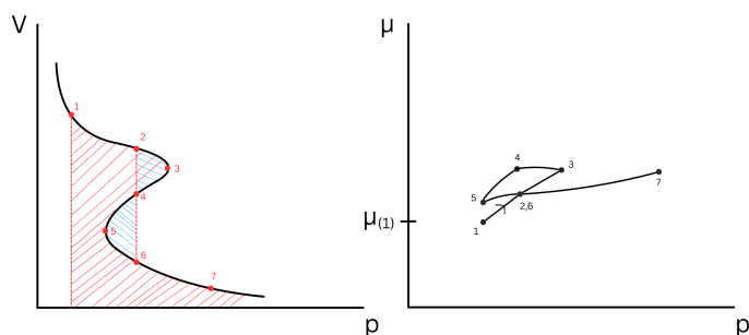
85. ábra. Kémiai potenciál ábrázolása Van der Waals-gáz esetén V - p grafikonon és a hozzátartozó \mu - p grafikonja
