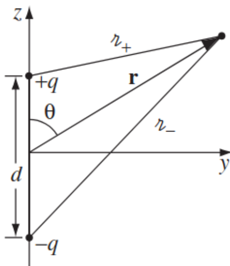
127. ábra. Elektromos dipólsugárzás geometriája
