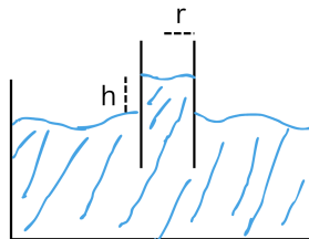
46. ábra. Kapilláris jelenség
