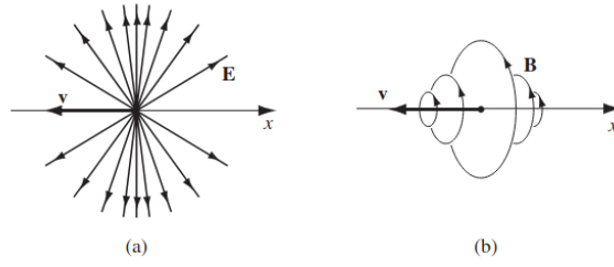
112. ábra. Mozgó töltés körüli elektromos és mágneses tér
