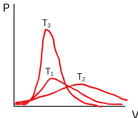
55. ábra. Kinetikus gázelmélet részecske sebesség eloszlása
