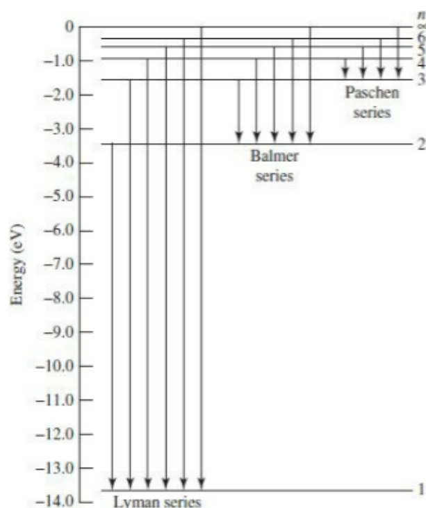
32. ábra. A Hidrogén atom spektrumának Energia szintjei és átmenetei.
