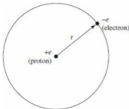
29. ábra. A Hidrogén atom
