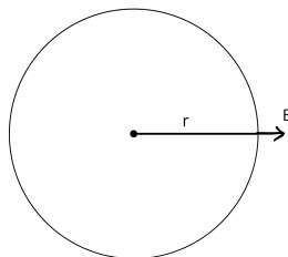
92. ábra. Gömbfelület ábrázolása
