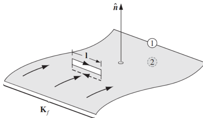
111. ábra. Gaussi hurok a felületen
