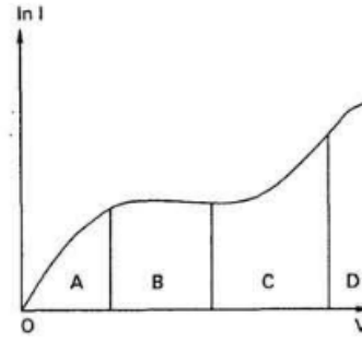
10.2. ábra. Ionizációs kamra feszültség-áram (V-I) karakterisztikája
