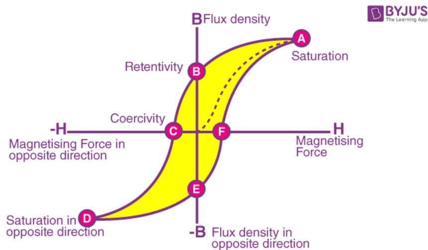
250. ábra. Hiszterézis-görbe egy ferromágneses anyag esetében.
