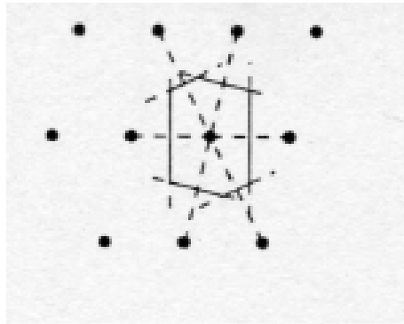
268. ábra. Wigner-Seitz cella egy 2D-s rács esetében.
