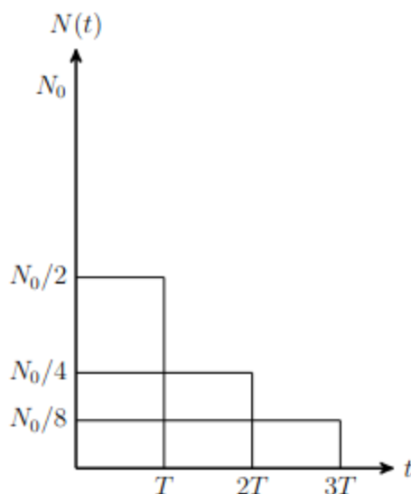
214. ábra. Exponenciális bomlástartörvény.
