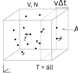
57. ábra. Kinetikus gázelmélet doboz modell
