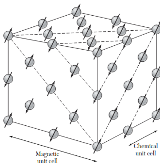
258. ábra. Antiferromágneses anyag illusztrációja.
