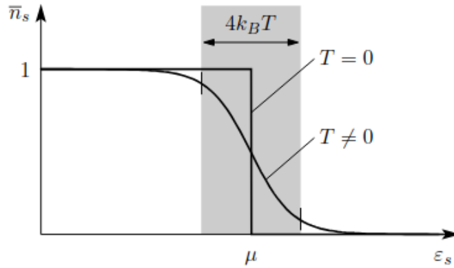
245. ábra. Fermi-Dirac eloszlás különböző hőmérsékleteken. Látható, hogy T \rightarrow 0 -nál az eloszlás lépcsőfüggvénnyé válik, ahol a kémiai potenciál megegyezik a Fermi-energiával.
