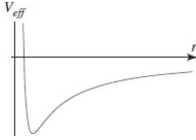
31. ábra. A Hidrogén atom effektív potenciálja
