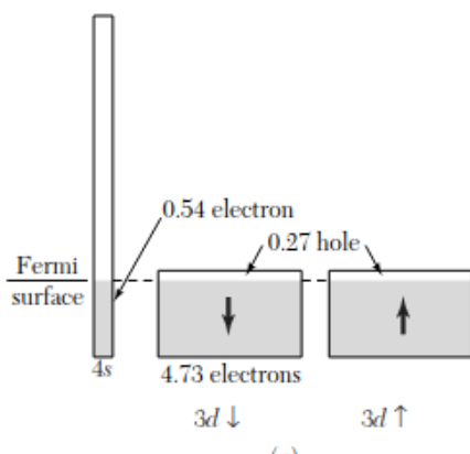
254. ábra. A Nikkel energiaszint diagramja T > T_C esetén.
