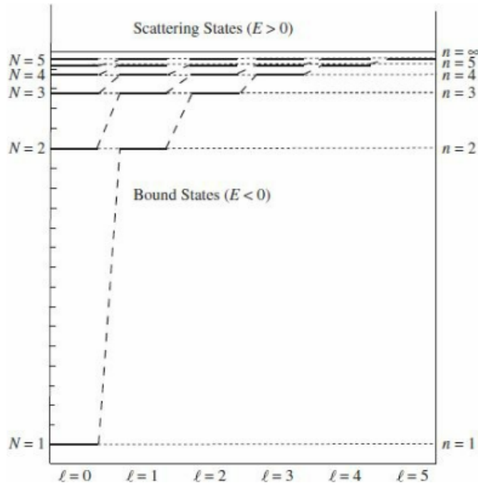
32. ábra. A Hidrogén atom energiaszintjei és hullámfüggvényei; n = 1 az alapállapot E_1 = -13.6 eV energiával; Végtelen számú állapot fér be n = 5 és n = \infty közé; E_\infty = 0 választja el a kötött és szabad állapotokat.
