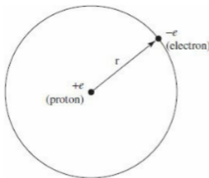
30. ábra. A Hidrogén atom
