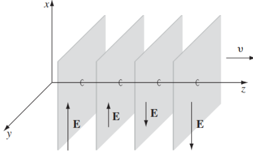
117. ábra. Planáris elektromágneses hullám vákuumban
