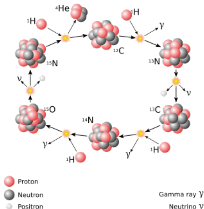
312. ábra. A CNO ciklus folyamata.
