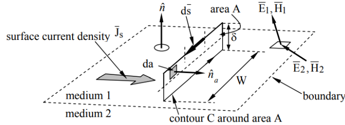
112. ábra. Gaussi hurok a felületen
