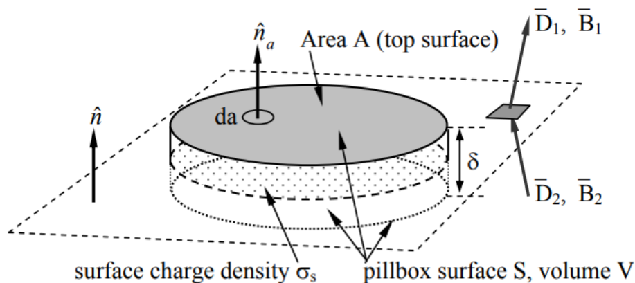
111. ábra. Egy "Gauss doboz" a felületen
