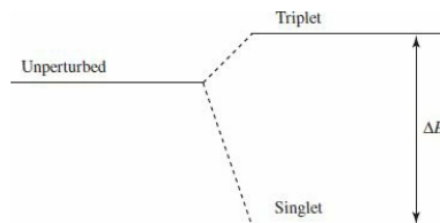
185. ábra. A Hidrogén atom alapállapotának hiperfinom felhasadása. A triplet állapot magasabb energiájú mint a szinglet állapot.
