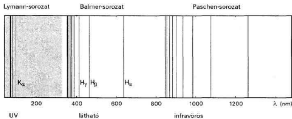
177. ábra. A hidrogénatom színeképe a hullámhossz függvényében. A ábrán három sorozat látható, az ultraibolya tartományban a Lyman-sorozat, a látható tartományban a Balmer-sorozat, az infravörös tartományban pedig a Paschen-sorozatot ábrázoltuk. A kísérletekben az egy sorozaton belüli egyre kisebb hullámhosszú vonalak intenzitása egyre csökken, ezért először a hidrogén 4 látható vonalát figyelték meg: H_\alpha, H_\beta, H_\gamma, H_\delta
