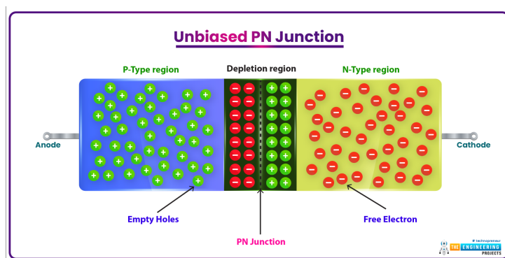
291. ábra. PN-átmenet felépítése és működési elve. A p-típusú és n-típusú félvezetők között egy határfelület jön létre, ahol a két anyag találkozik.
