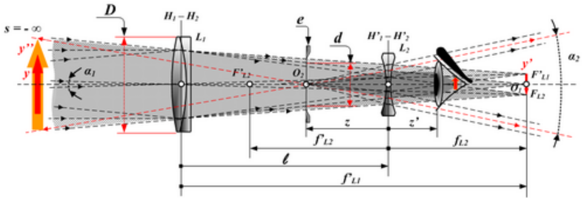
Figure 137: Galilei távcső felépítése: y - távoli objektum magassága, y' - valós kép magassága az objektívból, y'' nagyított kép magassága az okulárból, D - belépő pupilla magassága, d - virtuális kilépő pupilla, L_1 - objektív lencse, L_2 - okulár lencse, e - virtuális kilépő pupilla
