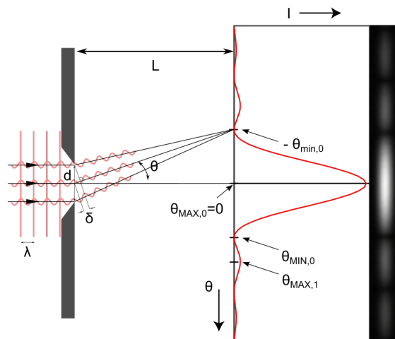
Figure 123: Diffrakció egy résen
