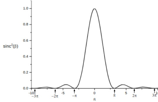
Figure 125: Diffrakciós intenzitás véges nyíláson
