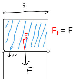
Figure 42: Felületi feszültség mérésének elve
