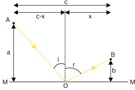
Figure 132: Fermat-elv visszaverődés esetén
