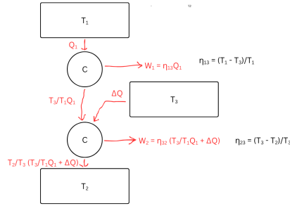
Figure 69: Carnot-gép schematikus ábrázolása több hőtartállyal
