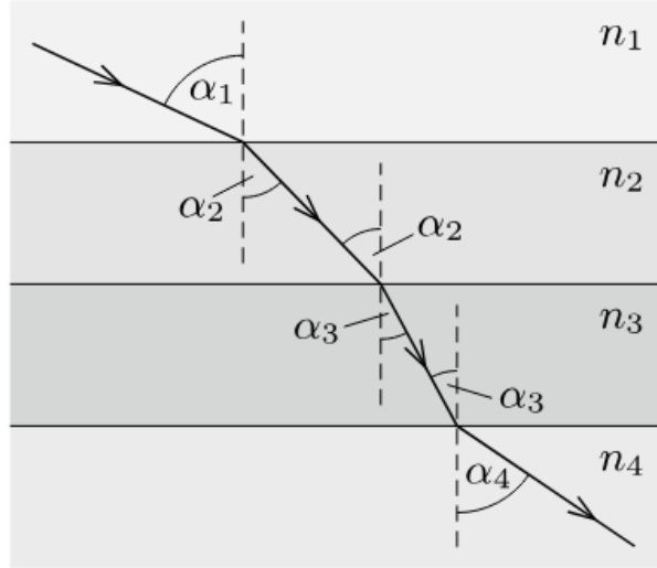
Figure 143: Délibáb kialakulása réteges levegőben
