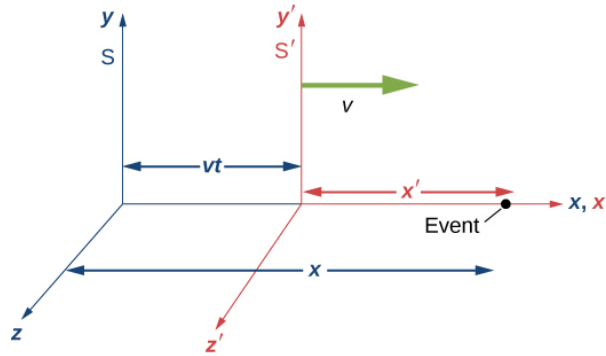
Figure 6: Lorentz transzformáció
