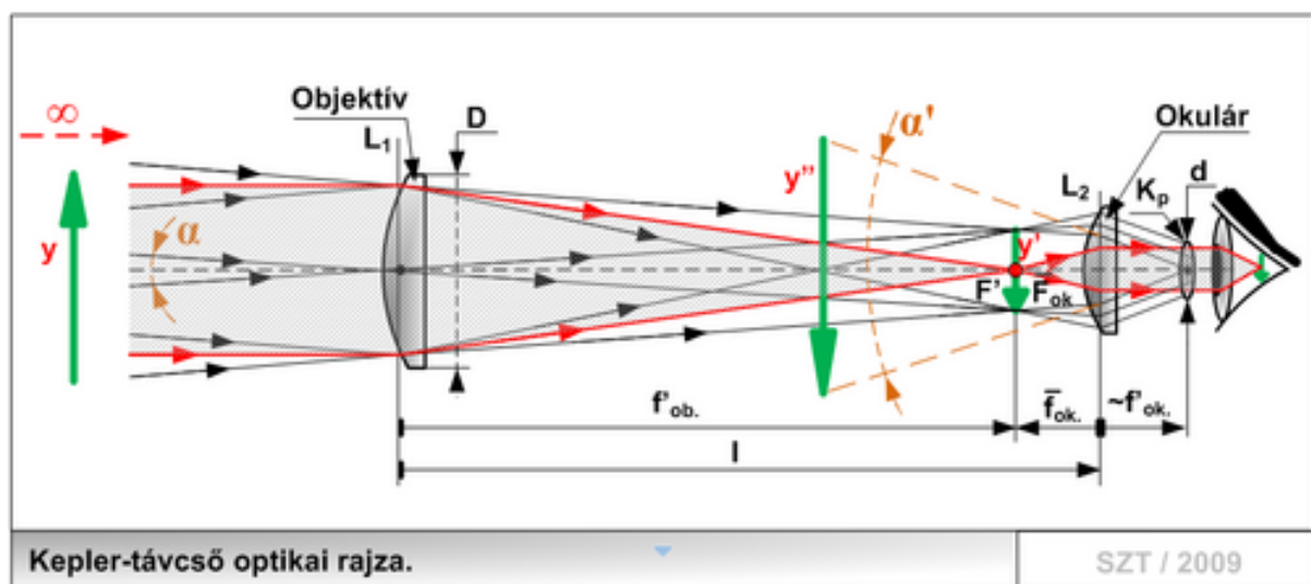
Figure 139: Kepler távcső felépítése
