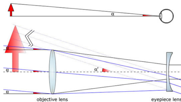
Figure 138: Galilei távcső fénypályája
