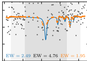
Ca II 8662
