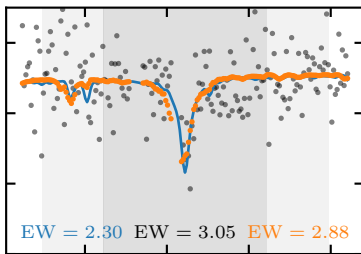
Ca II 8542
