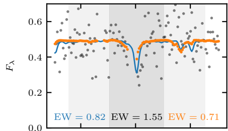
Ca II 8498
