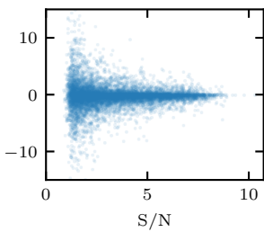
\Delta EW/EW TiO
