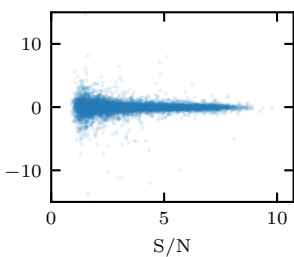
\Delta EW/EW Ca II 8542
