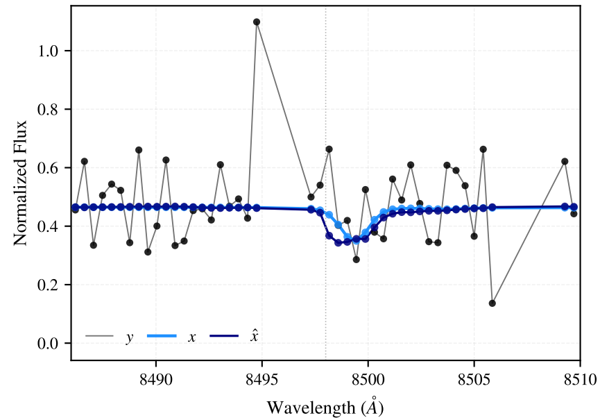
Ca II \lambda 8498
