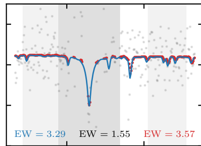
Ca II 8662
