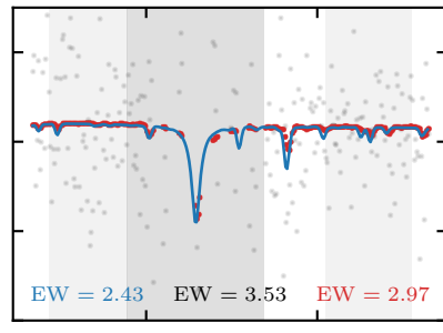
Ca II 8662
