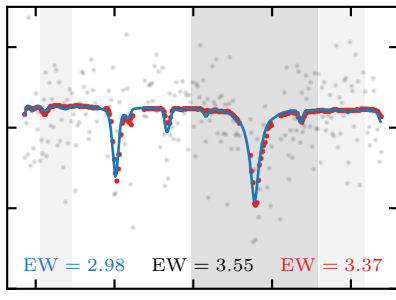
Ca II 8542
