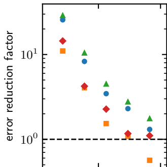
PCA
