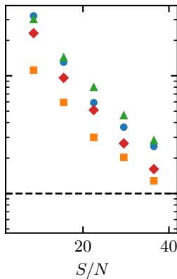
U-Net
