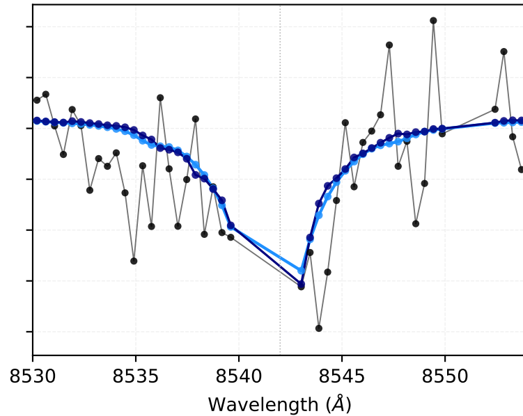
Ca II \lambda 8542
