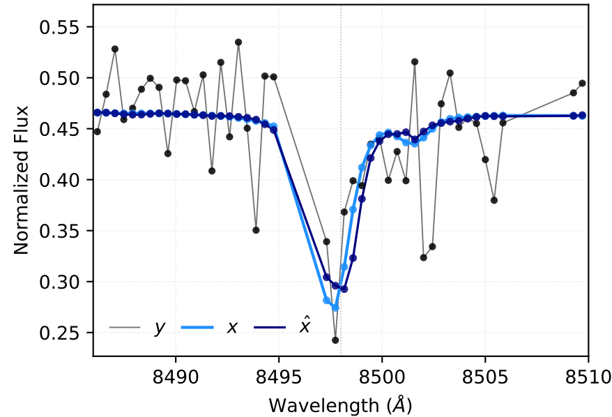
Ca II \lambda 8498
