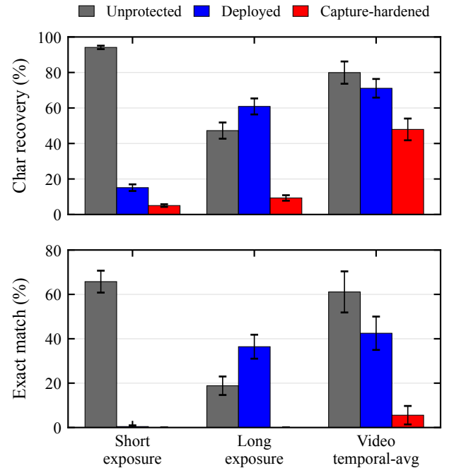
FIGURE 4. 真机防护效果: 档位 \times 攻击模式的 OCR 恢复率
