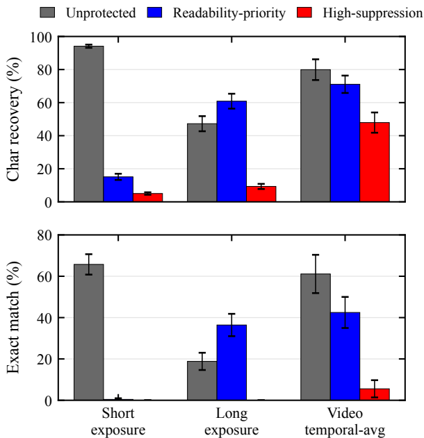
FIGURE 4. 三个代表性真机拍摄档位 (未保护、可读性优先和高抑制) 在短曝光、长曝光及 150 帧视频时域均值下的引擎最优 OCR 字符恢复率和完全匹配率, 汇总全部 9 个所测距离-角度配置。柱越低, 表示恢复出的文本越少。长曝光与视频柱揭示了积分边界: 即使可读性优先档的短曝光柱较低, 在积分攻击下仍保留大量可恢复内容。可读性优先档的样本数包含已披露的五项内容重复采集, 因此与其他档位不同。
