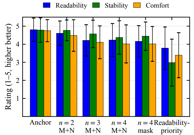
FIGURE 7. 六种评分显示条件下的可读性、稳定性和即时视觉舒适度的 1-5 级 Likert 平均评分 (误差线: 标准差), 条件从无掩蔽锚点排列至可读性优先完整配置。所有条目均为分值越高越好。
