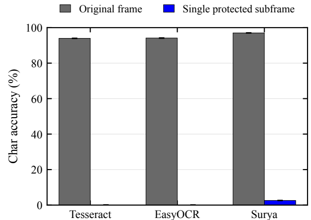
FIGURE 9. 三个 OCR 引擎在原始帧和单个受保护子帧上的字符恢复率; 误差线为以语料样本为单位重采样所得的 95% bootstrap 区间。
