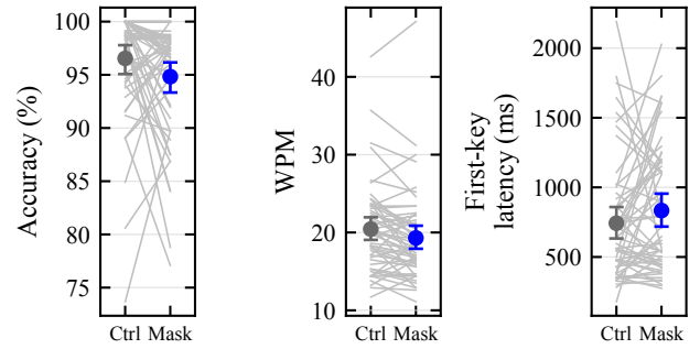
FIGURE 6. 控制条件与可读性优先掩蔽条件下的被试内打字表现: 每条灰线代表一名参与者 (每个条件下两次试验的均值); 标记表示组均值及参与者层面的 bootstrap 95% 置信区间。各面板依次显示转录准确率、每分钟词数和首次按键延迟。
