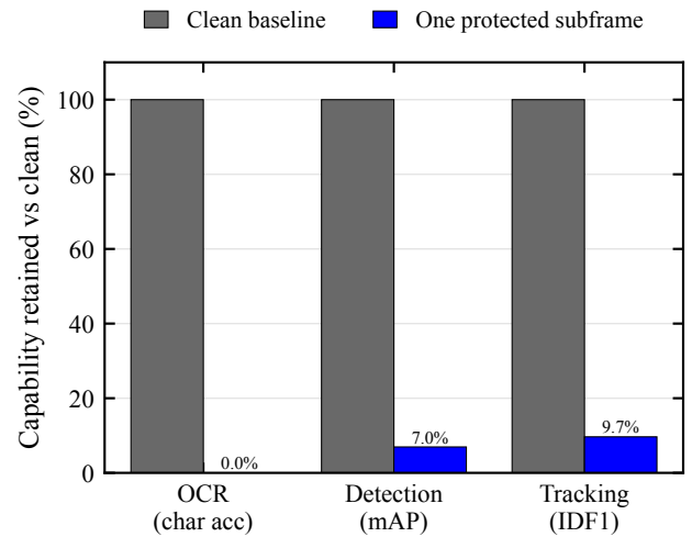
FIGURE 10. 评估的 OCR、检测和跟踪管线中，单个受保护子帧相对于干净基线（干净 = 100%）的剩余能力。各指标在任务内归一化，不可直接跨任务比较。
