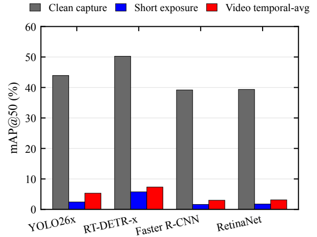
FIGURE 6. 四种检测器在未保护拍摄、短曝光受保护拍摄和 150 帧受保护均值下的真机 mAP50。各条件的保护、曝光、分辨率和帧约简方式不同。
