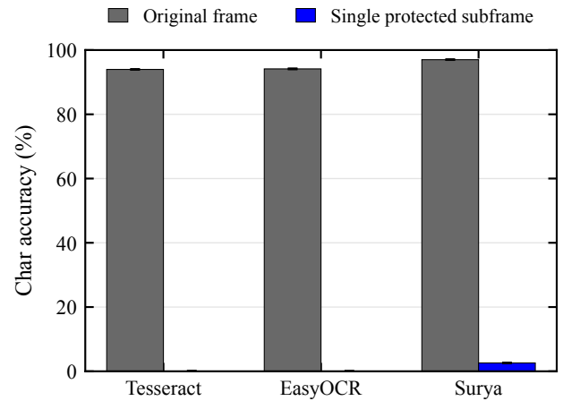
FIGURE 7. 三个 OCR 引擎在原始帧和单个受保护子帧上的字符恢复率; 误差线为以语料样本为单位重采样所得的 95% bootstrap 区间。
