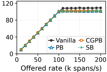
10 semconv
