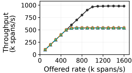
No semconv
