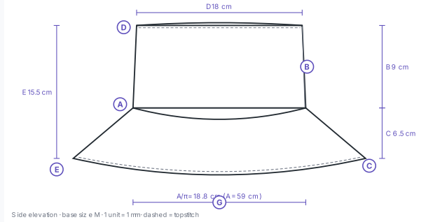
Side elevation · منظر جانبي
