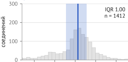
CYP1A2
