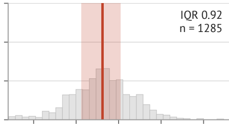
CYP2C9
