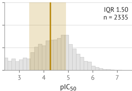
CYP3A4
