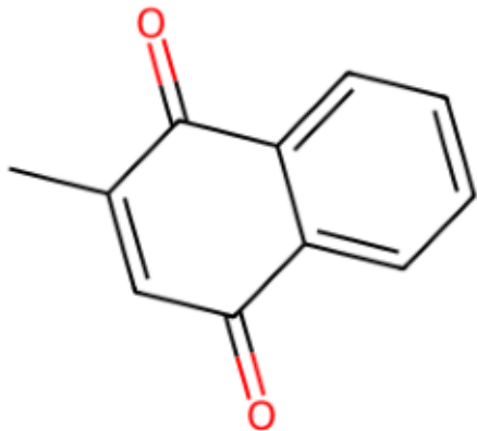
Vitamin K3
