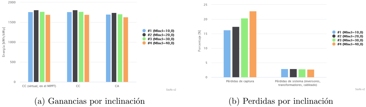
Figura 4: Repuesta del angulo de inclinación a la producción
