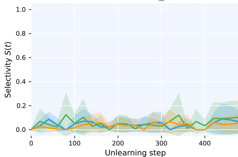
LunarLander no_tilt
