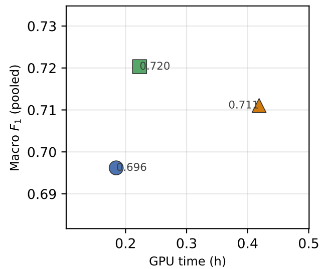
Qwen-3B
