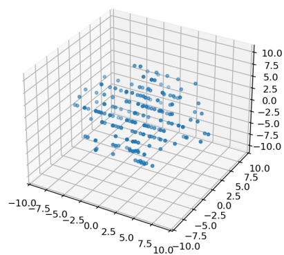
Default embedding
