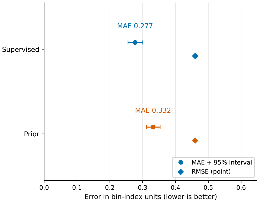
a Scalar ordinal error
