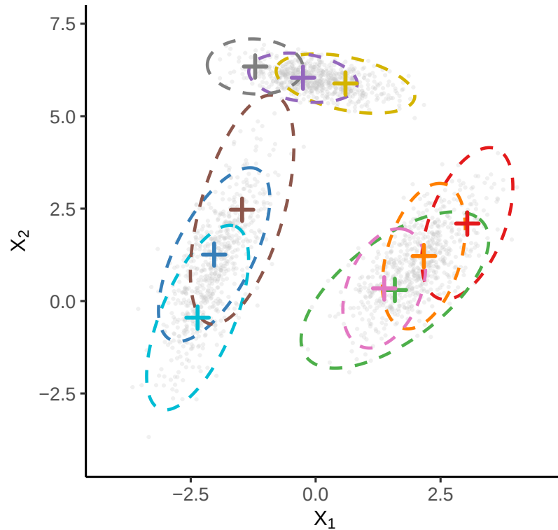
Overfitted MLE (k = 10)
