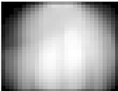
F6: T-shirt/top
