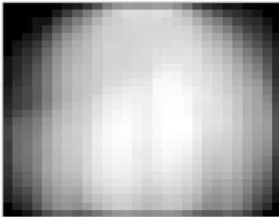
F10: Coat
