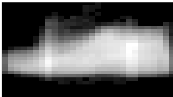
Vanilla NMF
