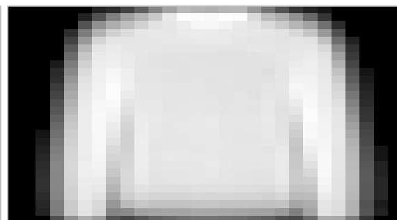
MiSo
