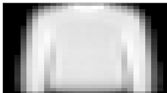
MiSo
