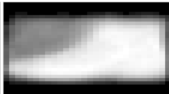
MiSo
