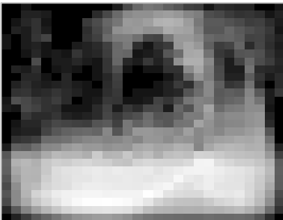
F13: T-shirt/top
