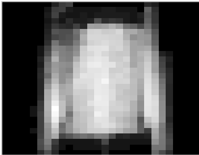
F11: T-shirt/top
