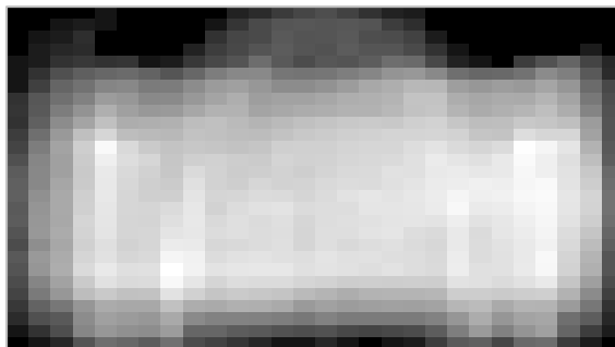
Vanilla NMF
