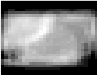
F18: Pullover
