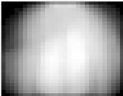
F15: T-shirt/top
