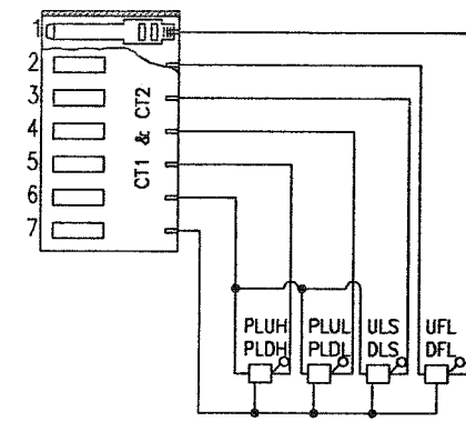
CT1&CT2 CONNECTION DIAGRAM (속도 90 M/MIN 이상)
