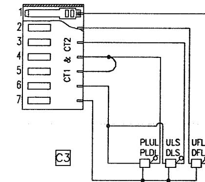
CT1&CT2 CONNECTION DIAGRAM (속도 60 M/MIN 이하)
