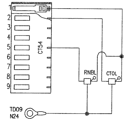
CT1&CT2 CONNECTION DIAGRAM (속도 90 M/MIN 이상)
