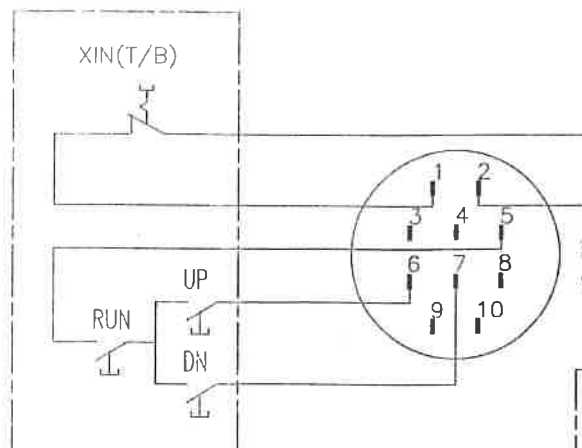
检修手柄接线示意图 INSPECTION HANDLE
