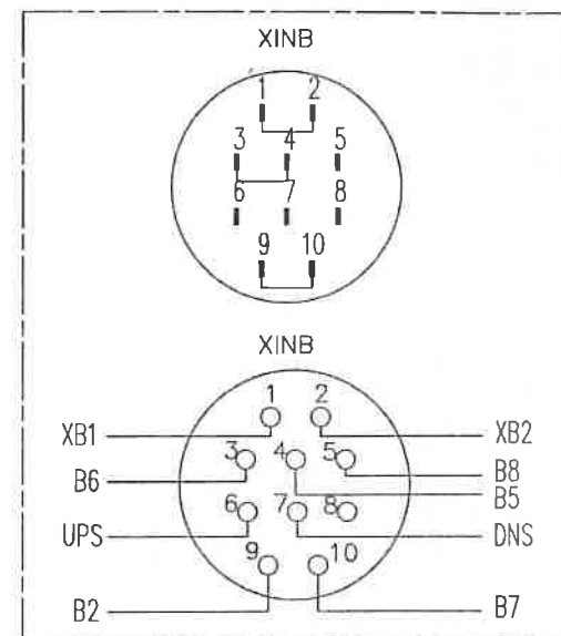
下检修手柄插座接线示意图 INSPECTION HANDLE SOCKET_BOT.
