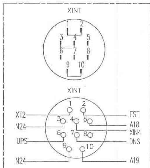
上检修手柄插座接线示意图 INSPECTION HANDLE SOCKET_TOP
