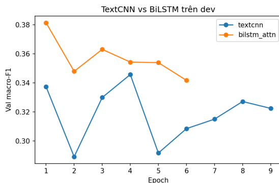
(a) TextCNN và BiLSTM trên validation
