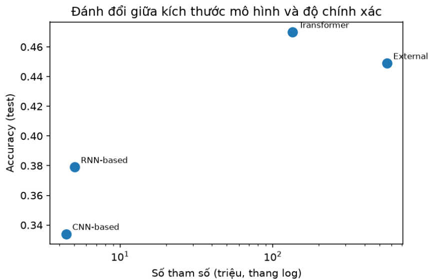
Hình 7.1: Đánh đổi giữa kích thước mô hình và độ chính xác
