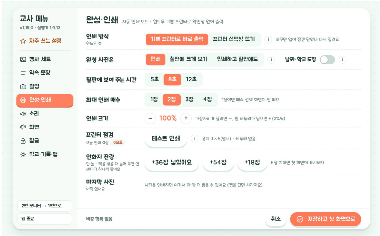
완성·인쇄 페이지.
