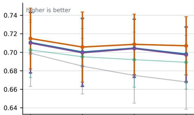
MAHNOB-HCI
