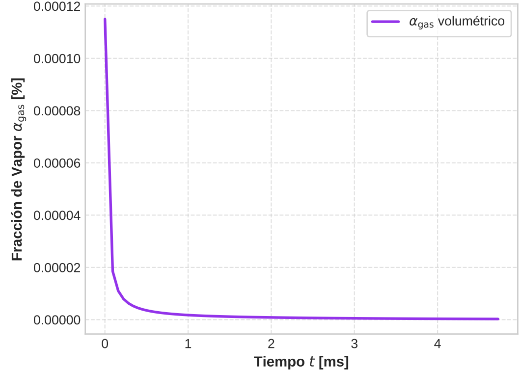
(d) Fracción de Fase Gaseosa (Cambio de Fase)
