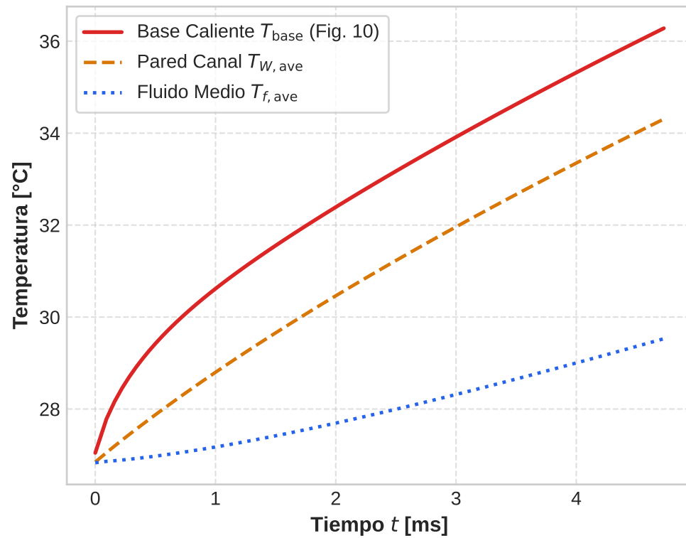
(c) Transferencia de Calor (Ecs. 11 y 12)
