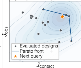
(d) Bayesian Optimization
