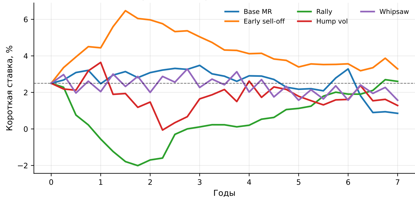
Пять stylized сценариев short rate в Hull-White
