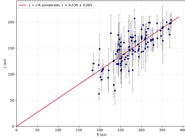
Figura 11: Ajuste lineal ponderado por mínimos cuadrados para el Grupo 2.
