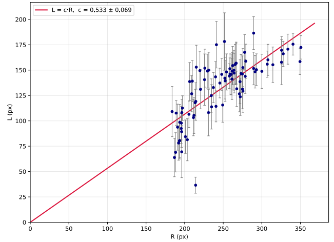
(b) Ajuste lineal para el grupo 1 con c = 0,533 .
