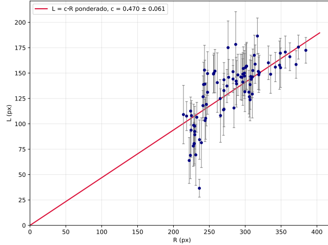
Figura 10: Ajuste lineal ponderado por mínimos cuadrados para el Grupo 1.
