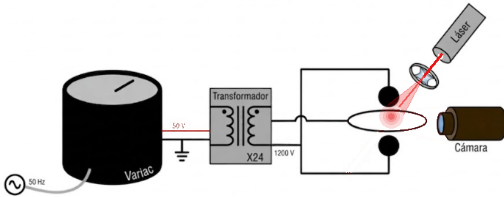
Figura 3: Esquema experimental de una trampa de Paul tridimensional, alimentando con 50 V a un transformador, se envía tensión al anillo de la trampa y a los electrodos por separado. Con un láser junto a una lente divergente se apunta al centro de la trampa, luego se graba allí, donde se colocan las partículas previamente cargadas.
