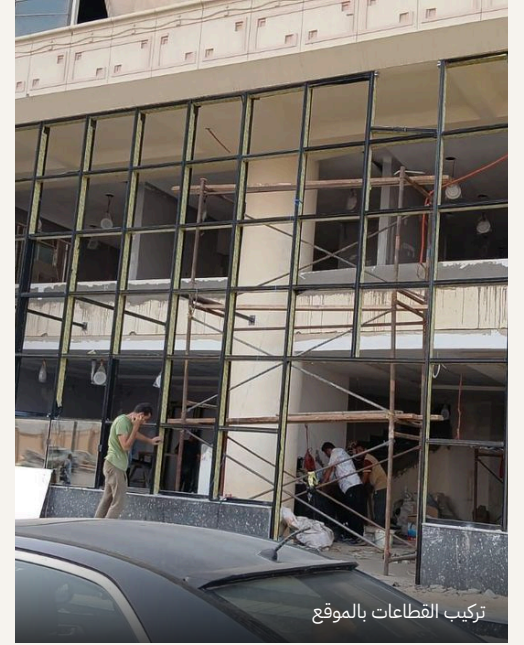
أعمال السقالات والتركيب
