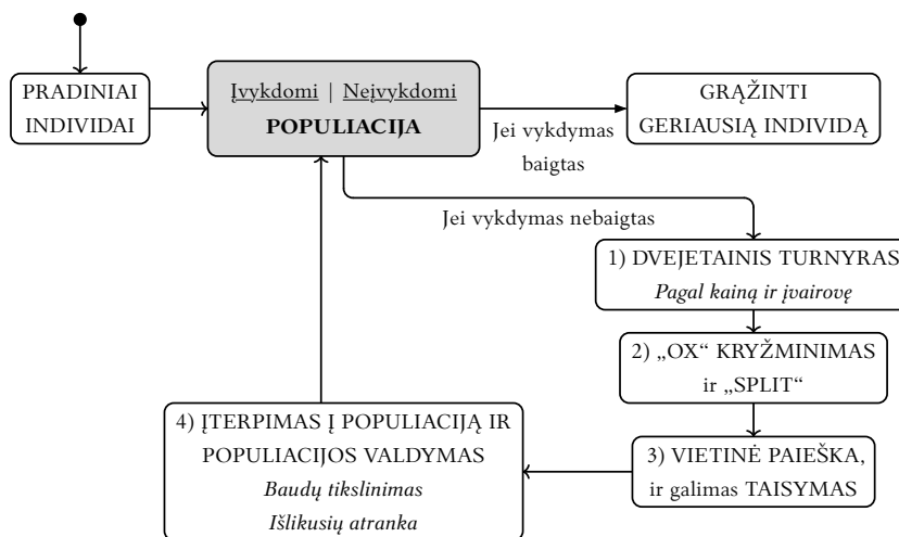
2 pav. HGS veikimas [Vid22]
