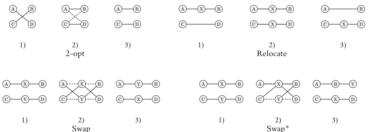
1 pav. Įvairių kaimynysčių veikimas
