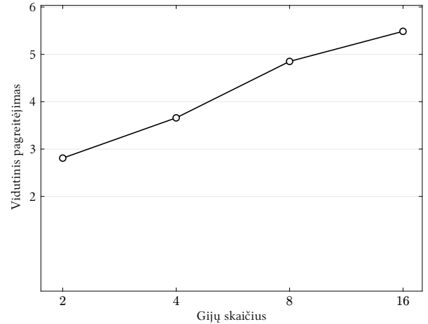
9 pav. Vidutinis pagreitėjimas, pasiektas skirtingu gijų skaičiumi. (Uchoa 2017 X-n rinkinys)
