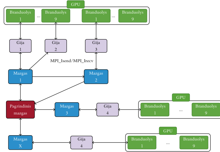
4 pav. Lygiagretintas HGS pagal [SND23]
