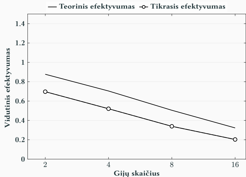
Pav. 6: Vidutinis ir tikrasis efektyvumas, (Uchoa 2017 X-n rinkinys)
