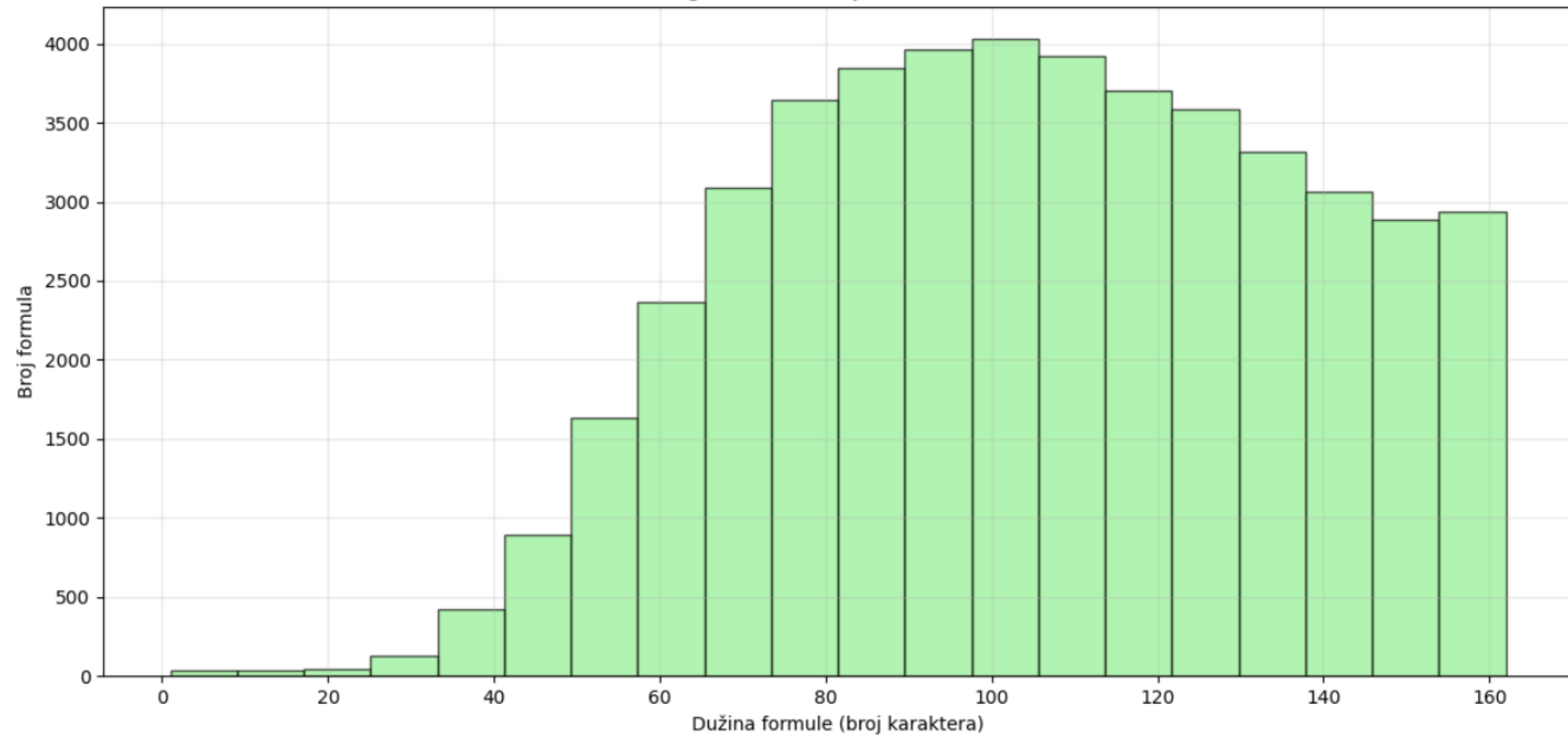
Histogram distribucije dužina formula
