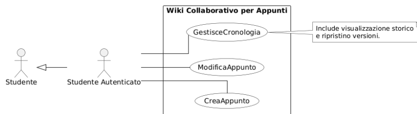
Figura 4.2: UC2 - Diagramma dei casi d'uso per l'attore Studente Autenticato
