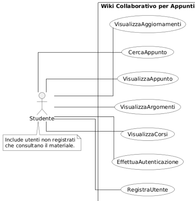
Figura 4.1: UC1 - Diagramma dei casi d'uso per l'attore Studente non autenticato
