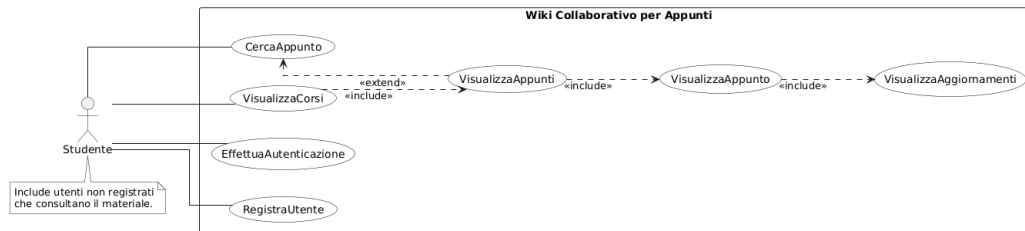
Figura 4.1: UC1 - Diagramma dei casi d'uso per l'attore Studente non autenticato
