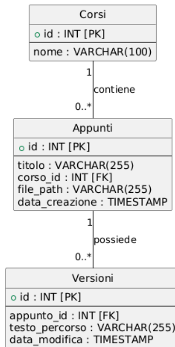
Diagramma ER - Schema Database Wiki
