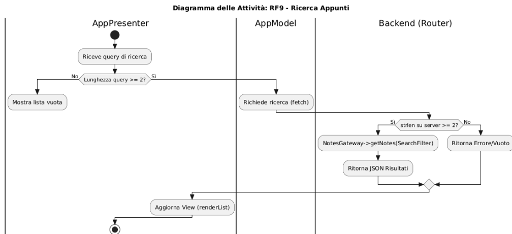
Figura 5.7: UC1 (RF9)
