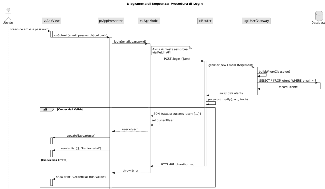
Figura 5.4: Login
