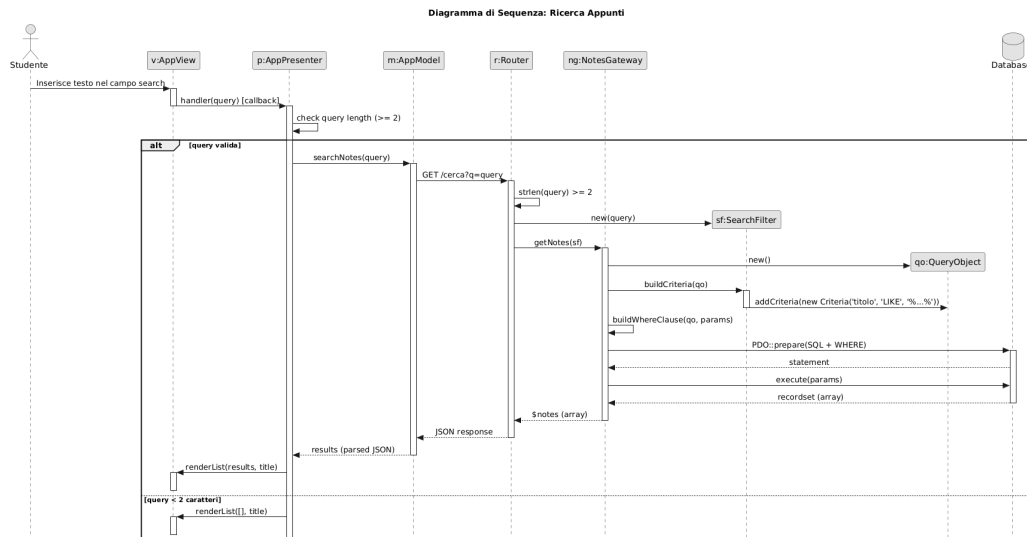
Figura 5.5: Ricerca Appunti
