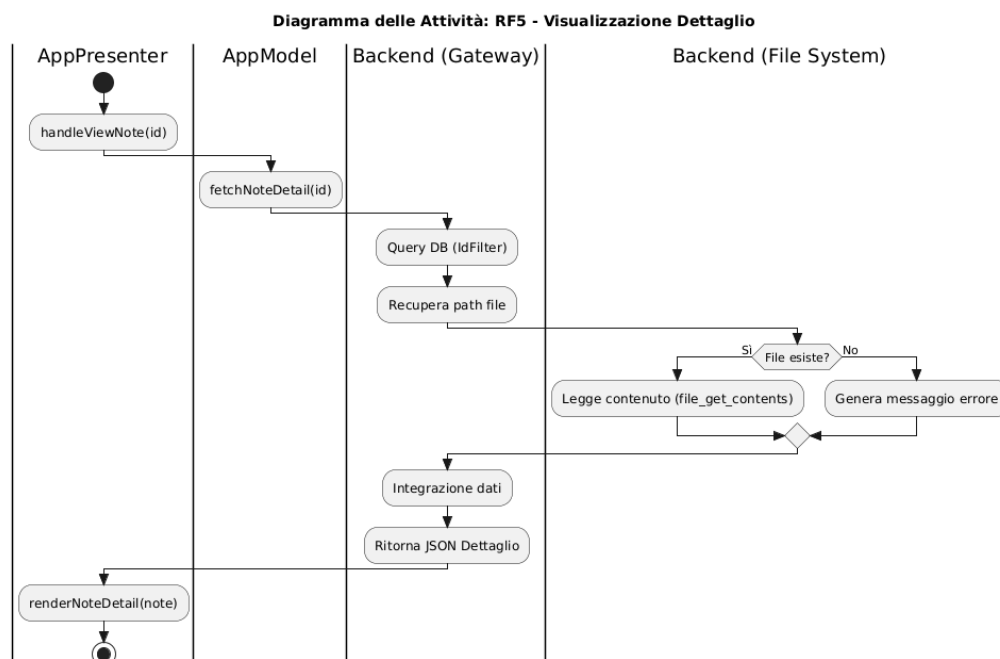
Figura 5.6: UC1 (RF5)
