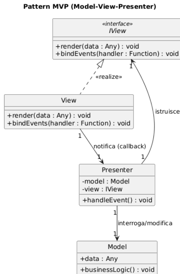
Figura 6.1: MVP
