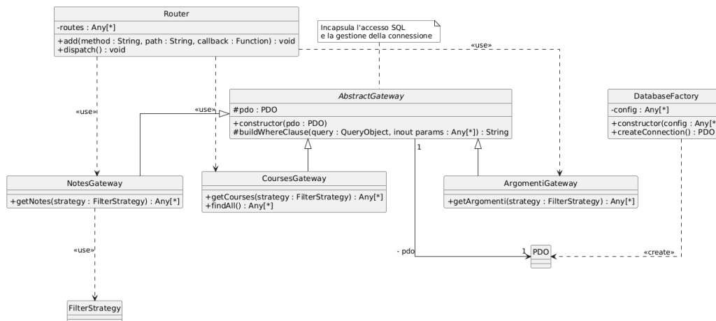
Figura 5.2: BE
