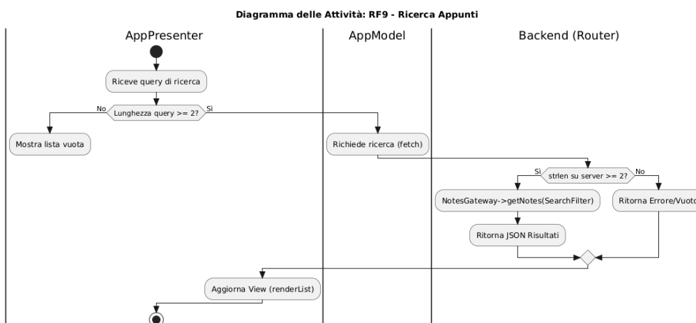
Figura 5.6: UC1 (RF9)
